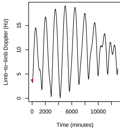
Doppler shift
